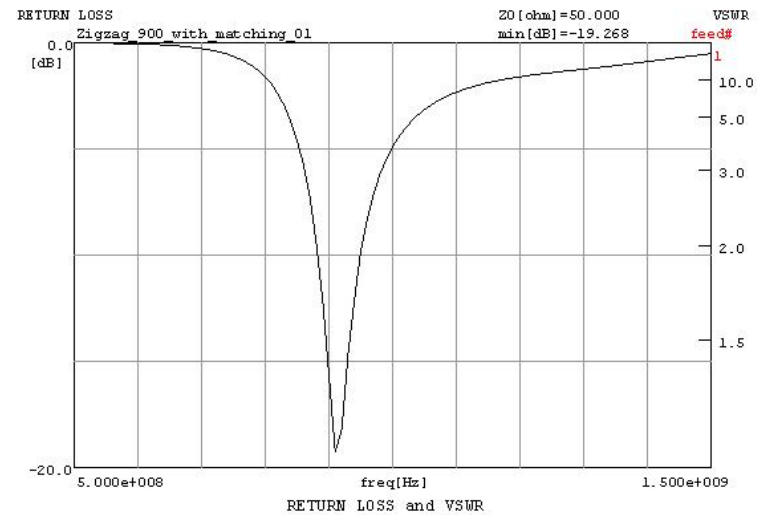
VSWR
